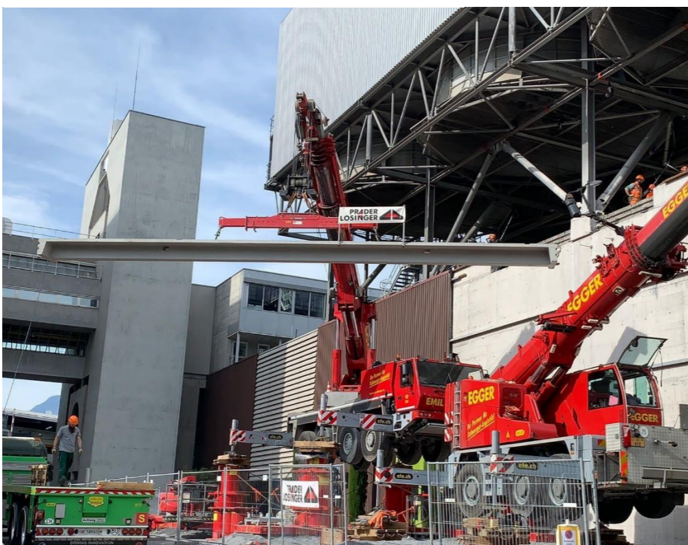
Montage des nouvelles poutres préfabriquées
