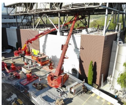
Vues d'ensemble de l'installation de chantier
